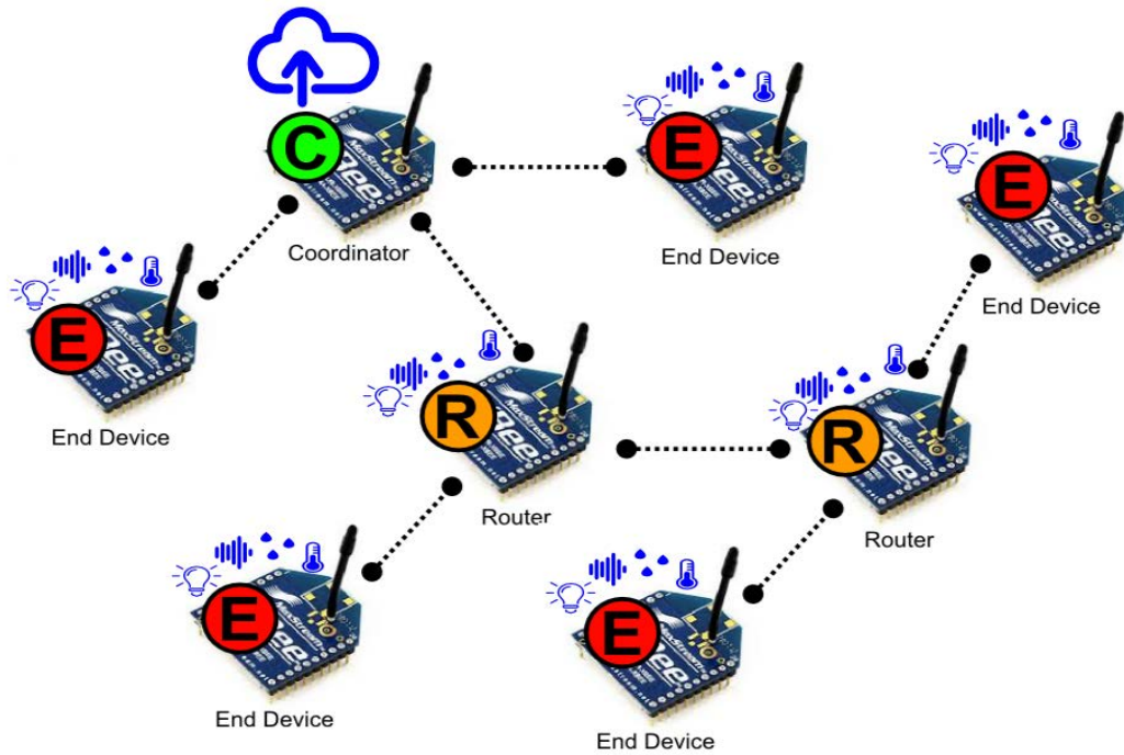
Figura 1 Arquitectura Red de sensores.
