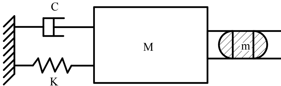
Figura 2.6.- Esquema de disipador de impacto de masa m (Soong y Dargush, 1997).
