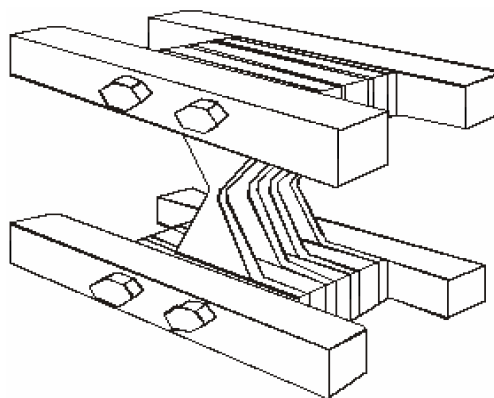
Figura 2.12 - Disipador metálico ADAS (Soong y Dargush, 1997).
