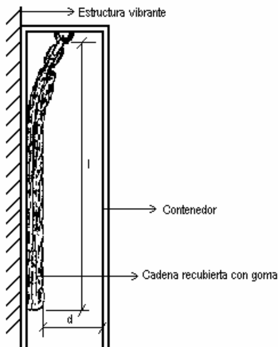
Figura 2.5.- Cadenas colgantes (Koss y Melbourne, 1995).
