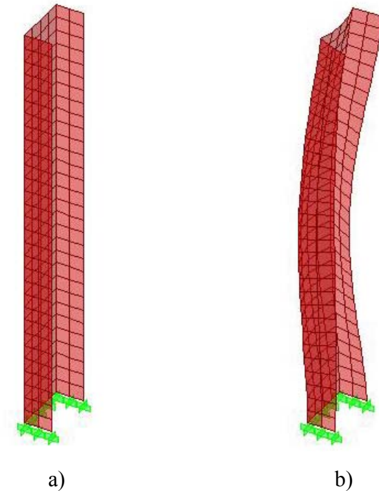
Figura 4.3 – Núcleo aislado. a) Modelo b) Segundo modo de vibración flexional
