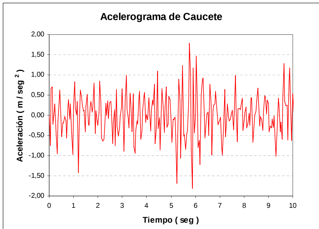
Figura 4.4 – Registros temporales de los acelerogramas usados en el núcleo aislado
