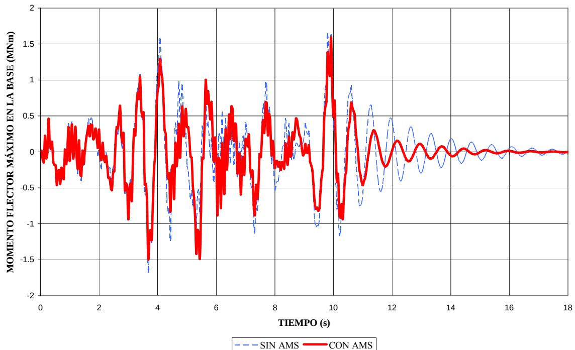
Figura 4.7 – Momento flector máximo en la base con y sin AMS. Sismo de Cauete.
