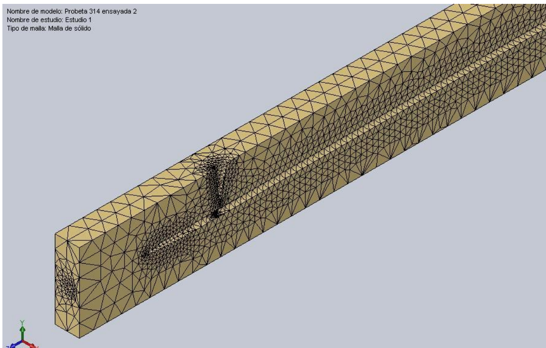
Figura 9 – Malla de elementos refinados en torno a los defectos
