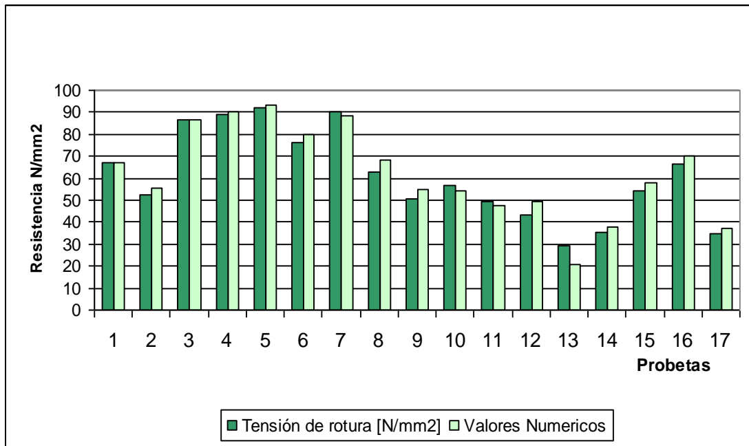
Figura 11 – Comparación de los valores empíricos y numéricos en la clase 1
