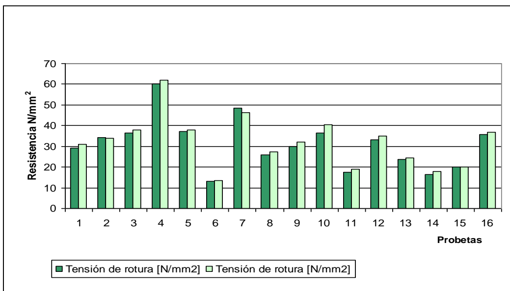
Figura 15- Comparación de los valores empíricos y numéricos en la clase 3
