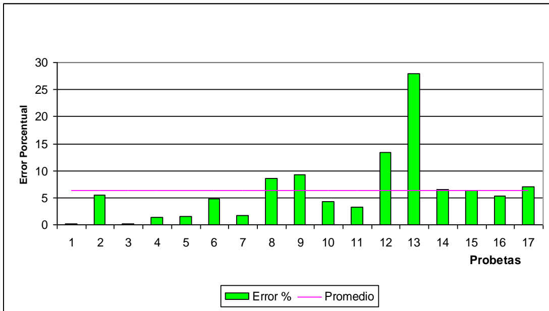
Figura 10 – Errores porcentuales de las probetas clase 1
