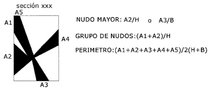
Figura 5 – Sección con nudosidad típica para explicar los criterios de evaluación de la nudosidad
