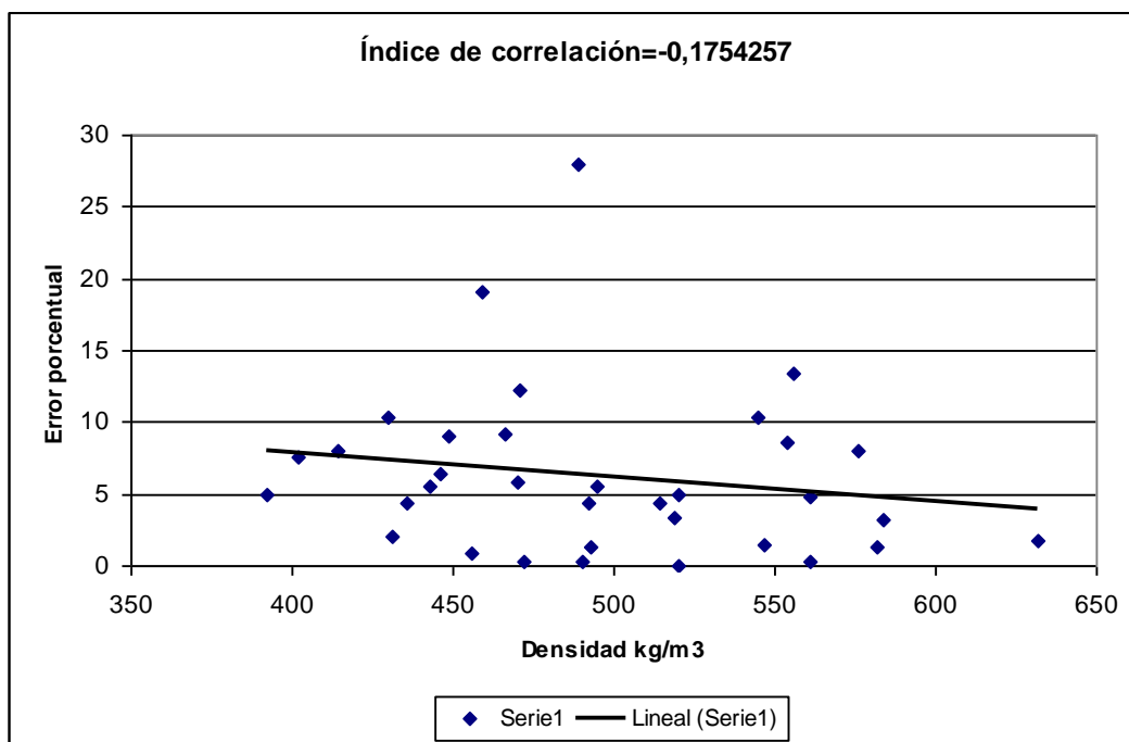
Figura 16 – Densidad versus error porcentual
