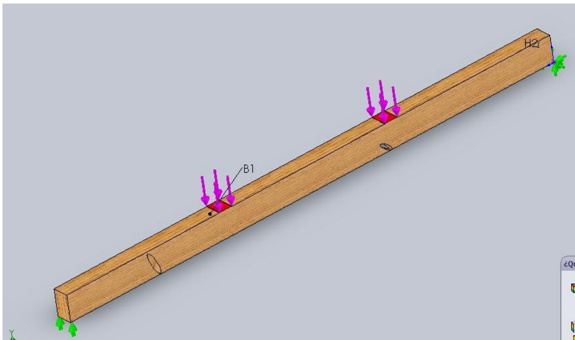
Figura 8 – Apoyos y cargas
