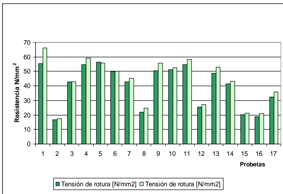
Figura 13- Comparación de los valores empíricos y numéricos de clase 2
