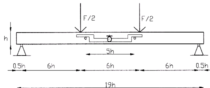
Figura 1: esquema de cargas para ensayo a flexión
