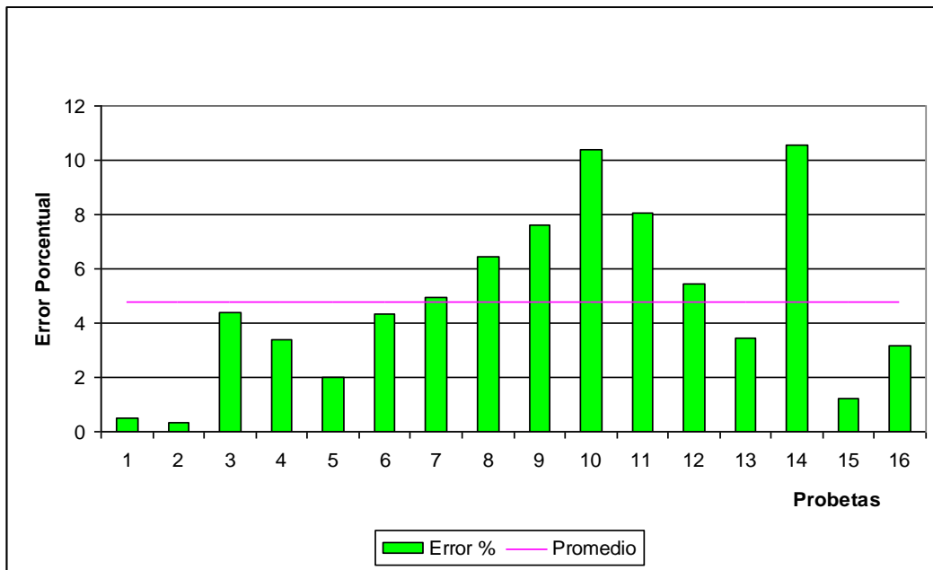
Figura 14- Error porcentual en probetas clase 3
