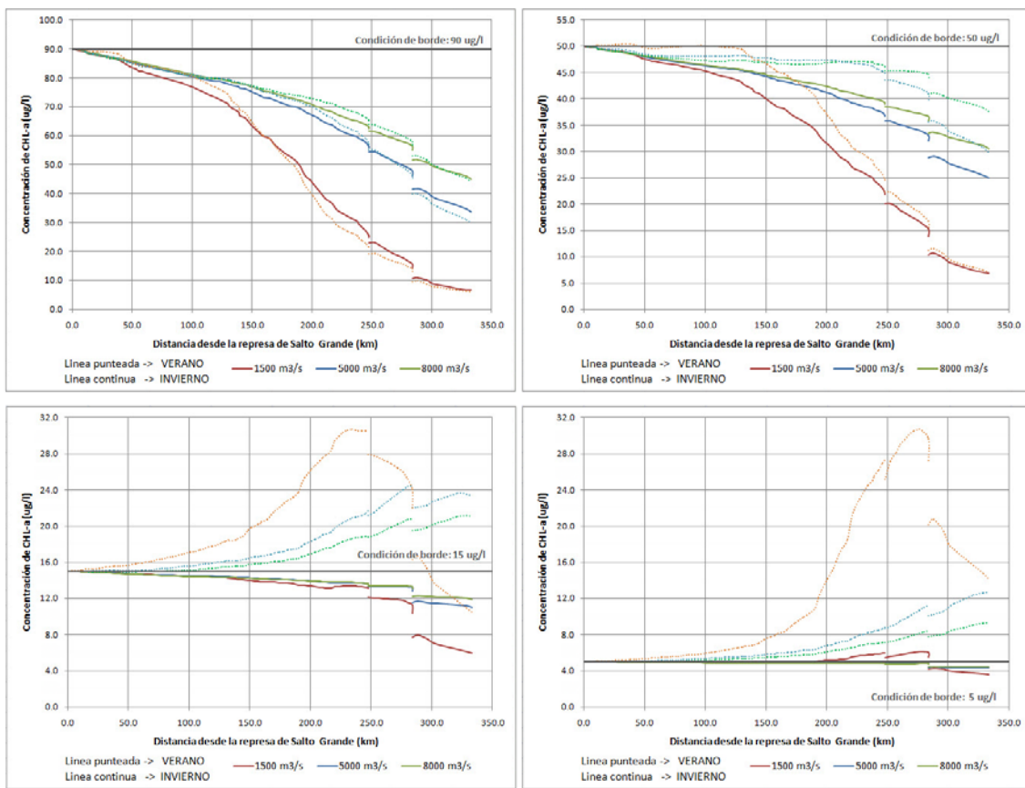
Figura 5. Concentraciones modeladas de Chl-a (µg/l) a lo largo del río Uruguay
