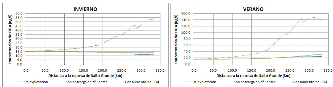
Figura 6. Concentraciones resultantes con aumento de PO 4 y con descarga de los afluentes, comparadas con las concentraciones resultantes correspondientes (antes simuladas), para invierno y verano
