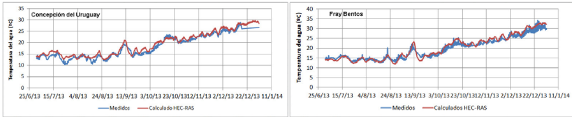
Figura 3. Temperatura del agua medida y calculada en Concepción del Uruguay y Fray Bentos
