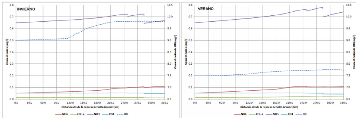
Figura 4. Concentraciones calculadas de NH4, Chl-a, NO3, PO4 y OD para las estaciones de invierno y verano, a lo largo del río Uruguay.
