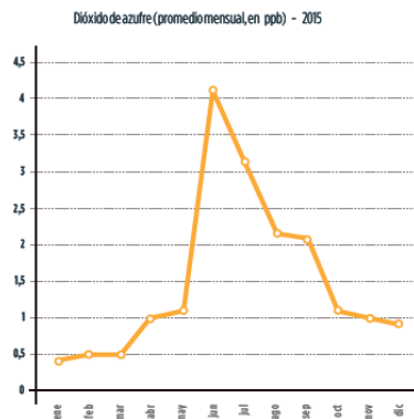
Figura 1. Medición de dióxido de azufre (SO 2 ) Promedio mensual en ppb, en Bahía Blanca (2015)
