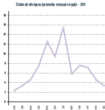
Figura 2. Medición de óxido de nitrógeno (NO x ) Promedio mensual en ppb, en Bahía Blanca (2015)
