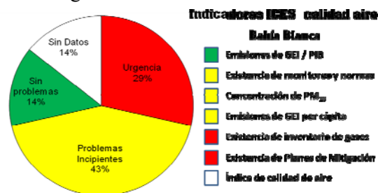
Figura 8. Indicadores ICES calidad de aire en Bahía Blanca.
