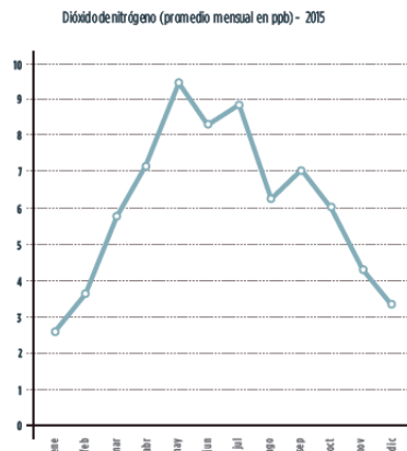
Figura 3. Medición de dióxido de nitrógeno (NO 2 ) Promedio mensual en ppb, en Bahía Blanca (2015)
