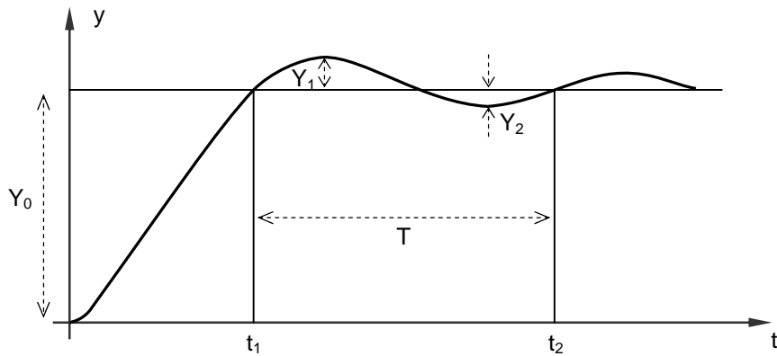
Fig. 2 Respuesta oscilante del sistema de segundo orden a la excitación de un salto escalón de amplitud Y_0
