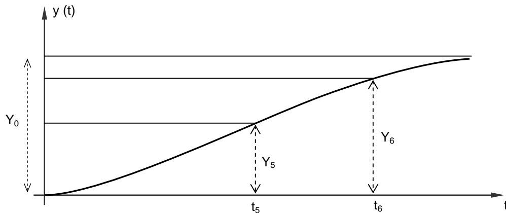
Fig. 4 Forma aproximada de la respuesta del sistema de segundo orden a la excitación de un salto escalón de amplitud Y_0 cuando el valor de \zeta es mayor que 2.
