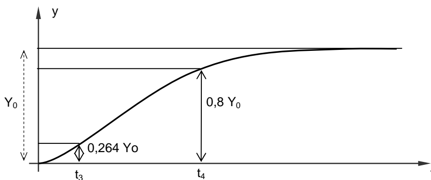
Fig. 3 Forma aproximada de la respuesta del sistema de segundo orden a la excitación de un salto escalón de amplitud Y_0 cuando el valor de \zeta está comprendido entre 0,5 y 2.
